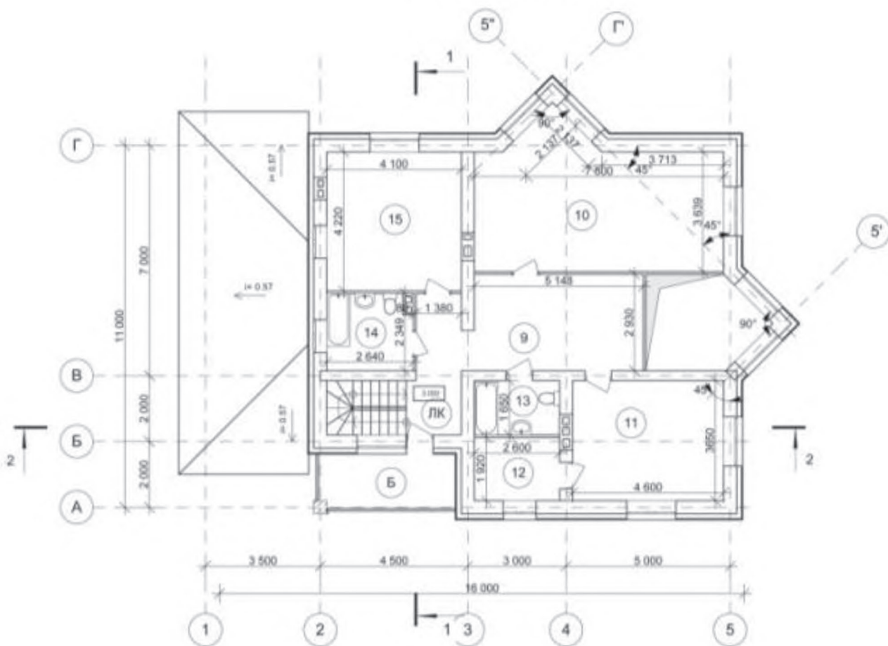
Экспликация 2 этажа
